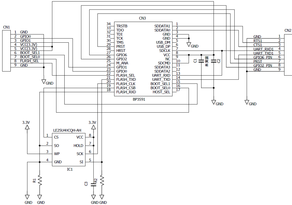
図 4 BP359D 回路図
