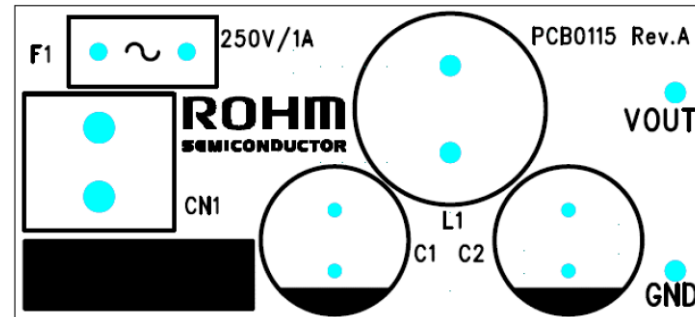
Top Layer
