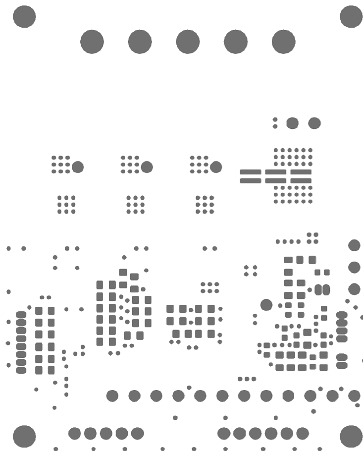
Bottom_Mask
