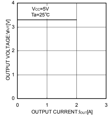
Fig.5 Iout-Vout
