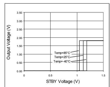
Fig. 45. STBY Threshold
