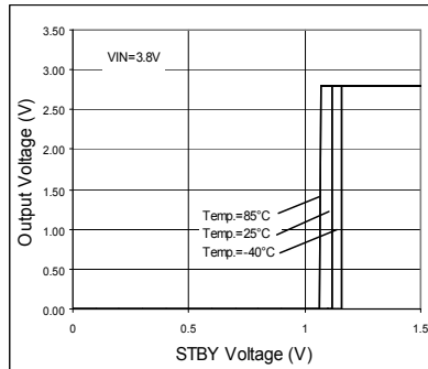
Fig. 10. STBY Threshold
