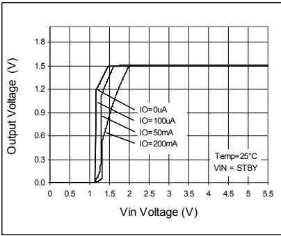
Fig. 66. Output Voltage
