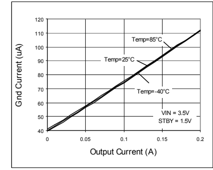
Fig. 42. IOUT - IGND
