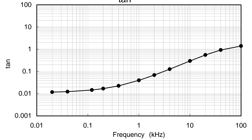
tan
