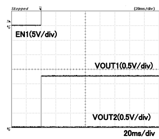
VIN=5.5V,EN2=L(OFF)
