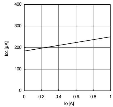
Fig.30 IO-ICC
