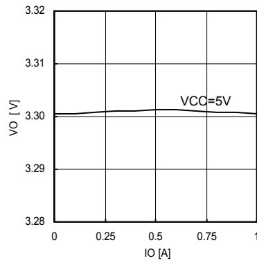
Fig.17 IO-VO (VO=3.3V)
