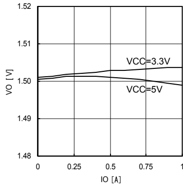
Fig.14 IO-VO (VO=1.5V)
