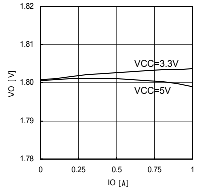
Fig.15 IO-VO (VO=1.8V)
