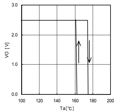
Fig.19 TSD (IO=0A)
