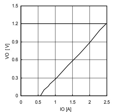
Fig.24 OCP (VCC=5V, VO=1.2V)
