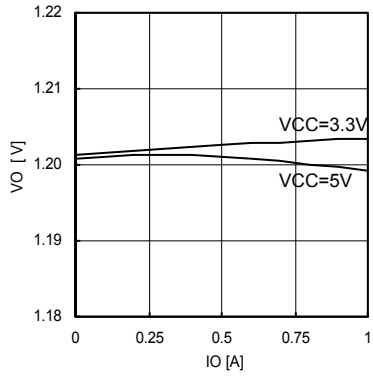
Fig.13 IO-VO (VO=1.2V)
