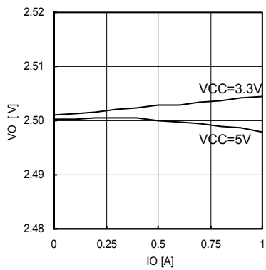
Fig.16 IO-VO (VO=2.5V)
