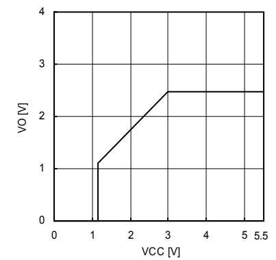
Fig.18 VCC-VO (IO=0A)
