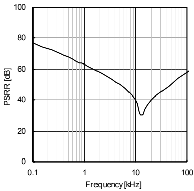
Fig.31 PSRR(IO=0A)
