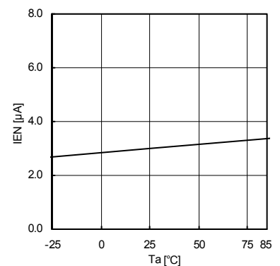
Fig.12 Ta-IEN
