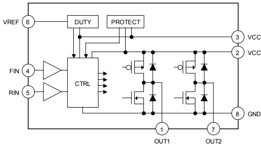
Fig.1 BD6230F / BD6231F
