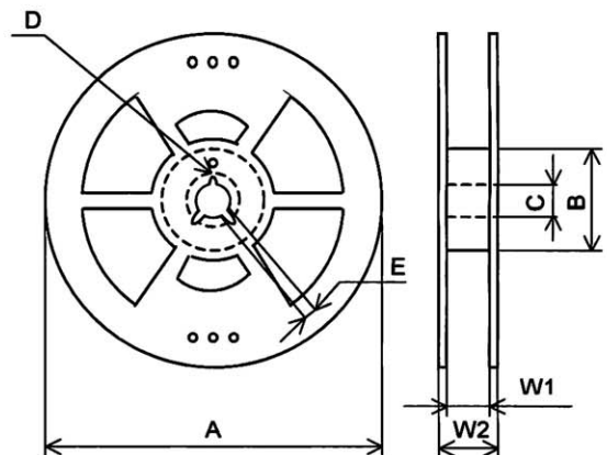
Fig. 4 Reel dimensions
