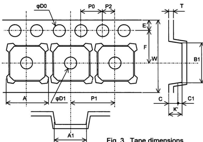
Fig. 3 Tape dimensions
