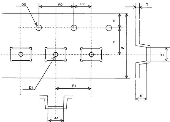
Fig. 3 Tape dimensions
