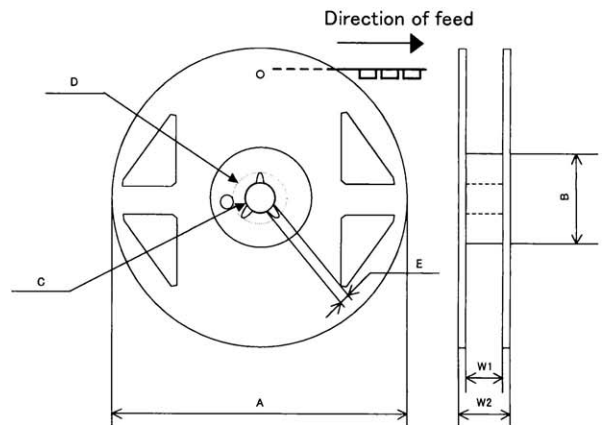
Fig. 4 Reel dimensions
