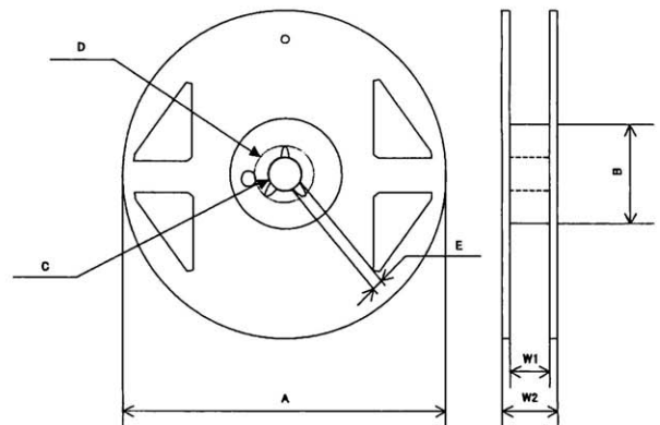
Fig. 4 Reel dimensions
