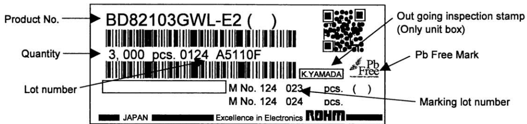
Fig. 5 Label example
