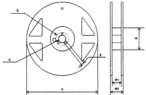
Fig. 4 Reel dimensions
