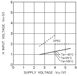
Fig. 2 H input voltage V_H (CS,SK,DI)
