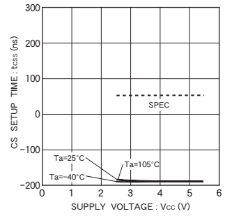
Fig. 19 CS setup time t_{cSS}
