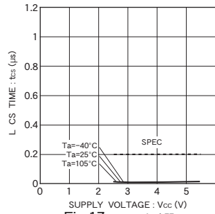
Fig. 17 CS setup time t_{cS}
