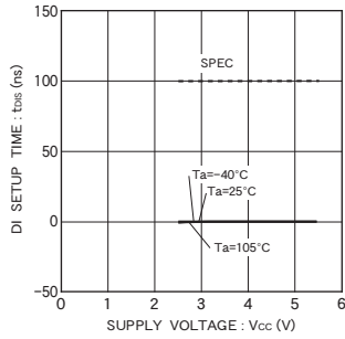
Fig. 21 DI setup time t_{dIS}
