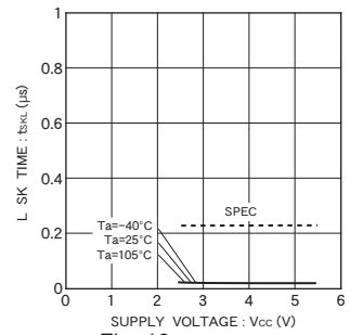
Fig. 16 SK low time t_{sKL}
