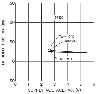
Fig. 20 DI hold time t_{dIH}
